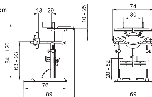
STANDY 3 medio - Peso 28,9 kg - Capacidad Máx. 90 kg
