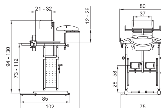
STANDY 4 grande - Peso 38 kg - Capacidad Máx 120 kg
