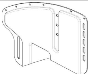
YNG040201 Protector aluminio sin fender
