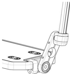
YNG050108 Mecanismo para abatir la plataforma
